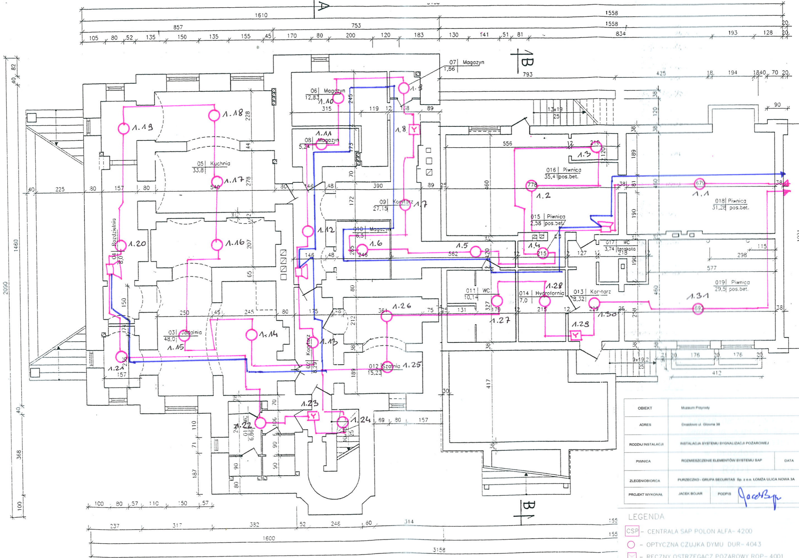
RZUT PIWNIC skala 1:100
